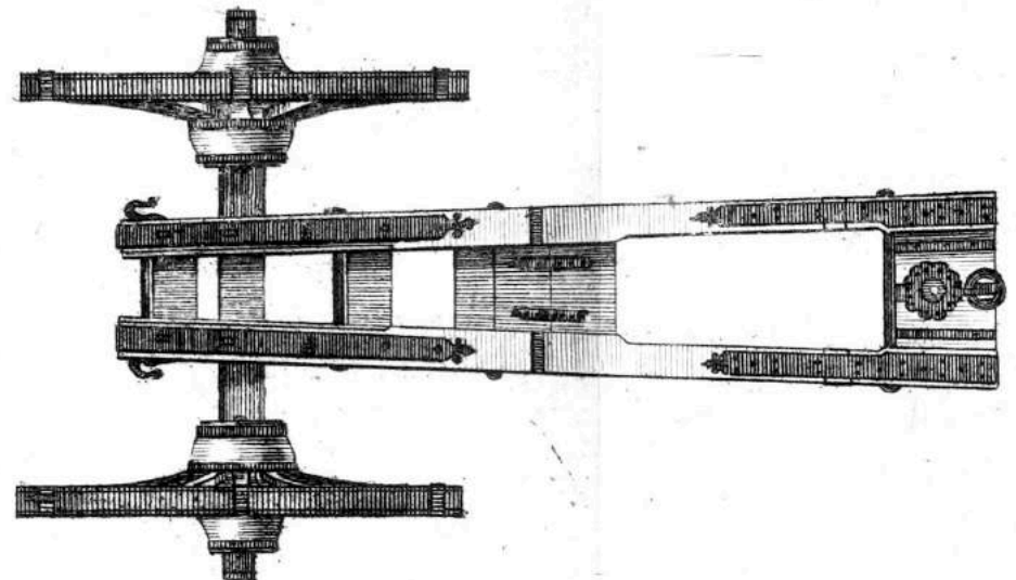
6 pond kanon – Mémoires d'artillerie – Surirey de Saint-Remi
