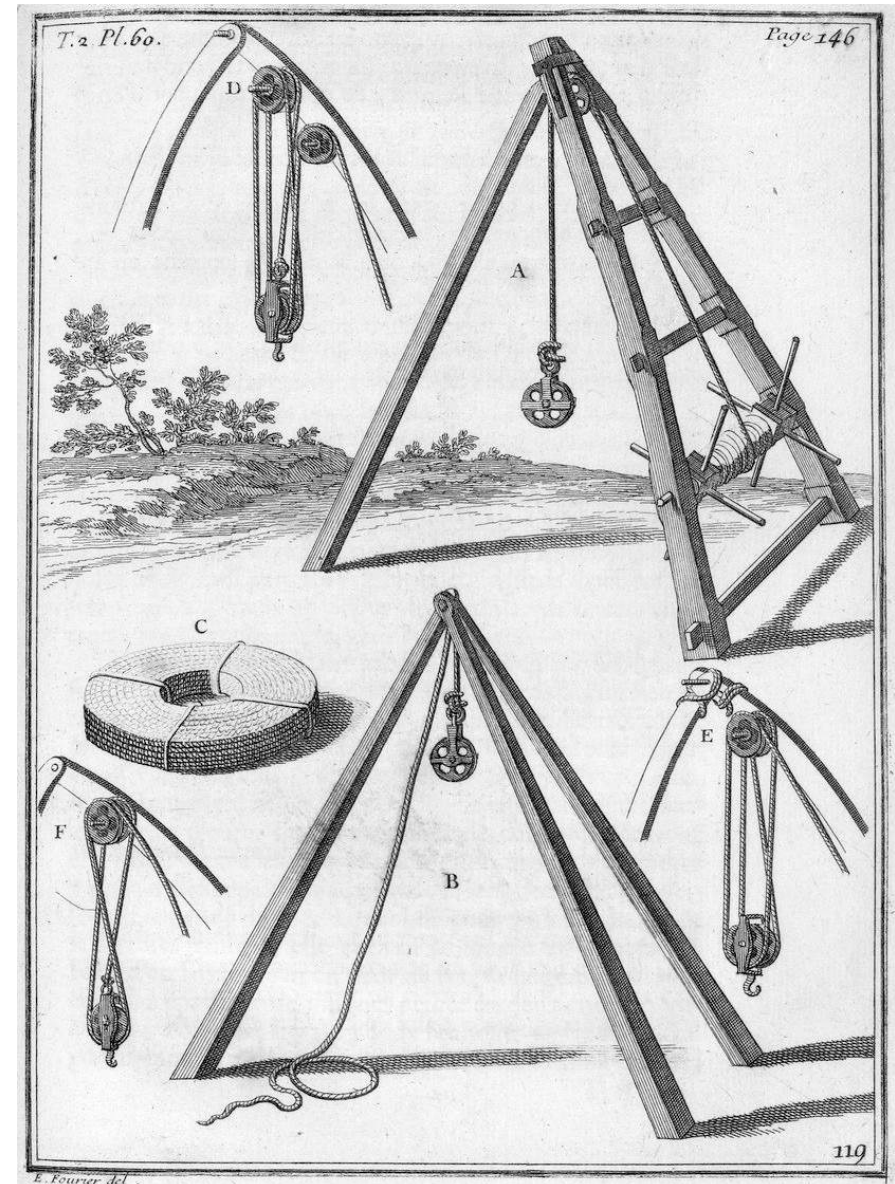
Monteren van een kanonsloop op een affuit (17de eeuw)
