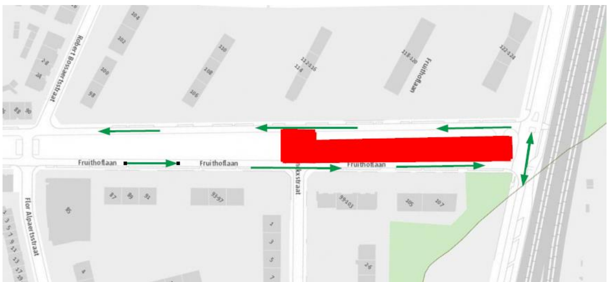
Fase 2b (rood is werfzone)
